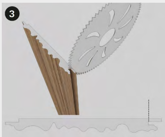
3 Tagliare il nuovo pannello come mostrato in figura, eliminando il labbro dell'incastro "femmina".
